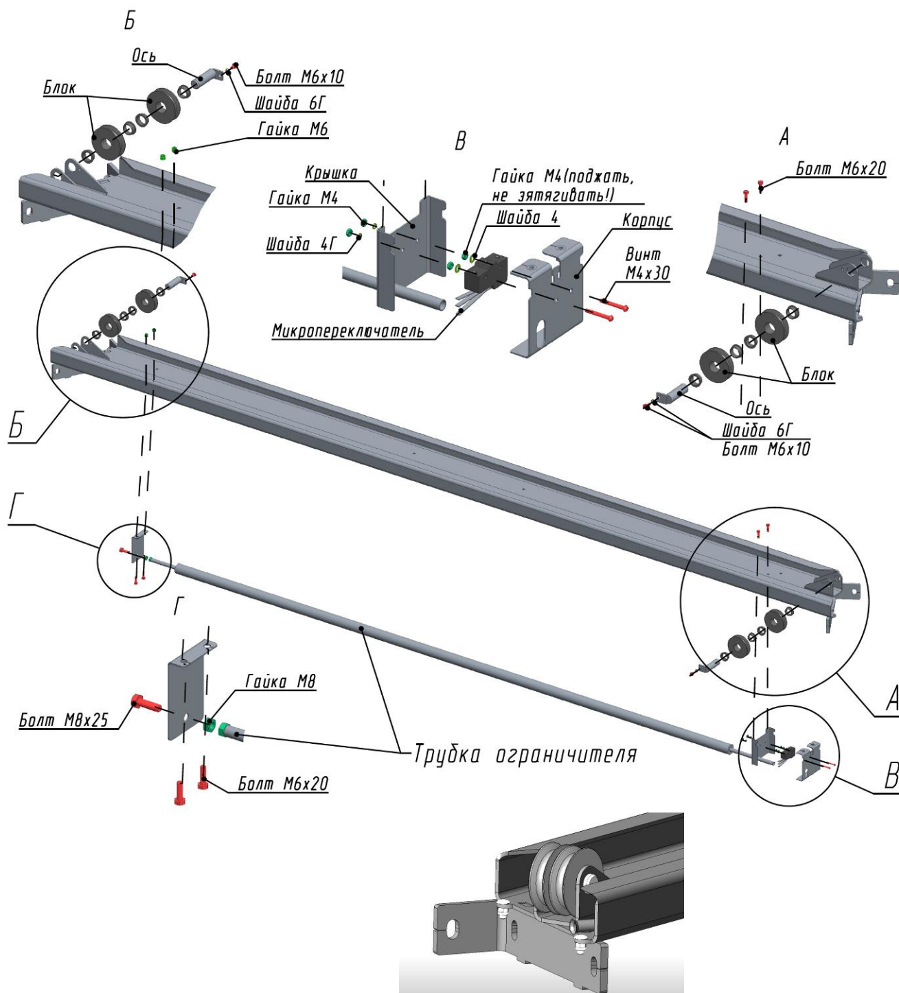
Рисунок 6.2.1 – Сборка перекладины
